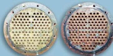
實證二：充滿水垢的冷凝器
